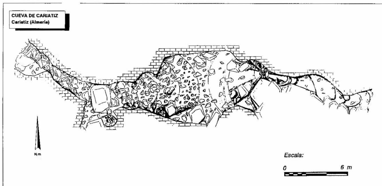
Figura 4 Cueva Cariatiz (Cariatiz, Almería). Topografía: (F. Risco, SECAM)
