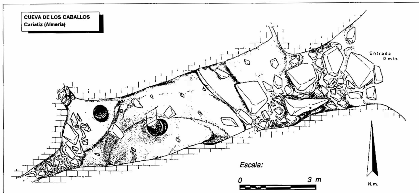
Figura 2 Cueva de los Caballos (Cariatiz, Almería). Topografía: (F. Risco, SECAM)
