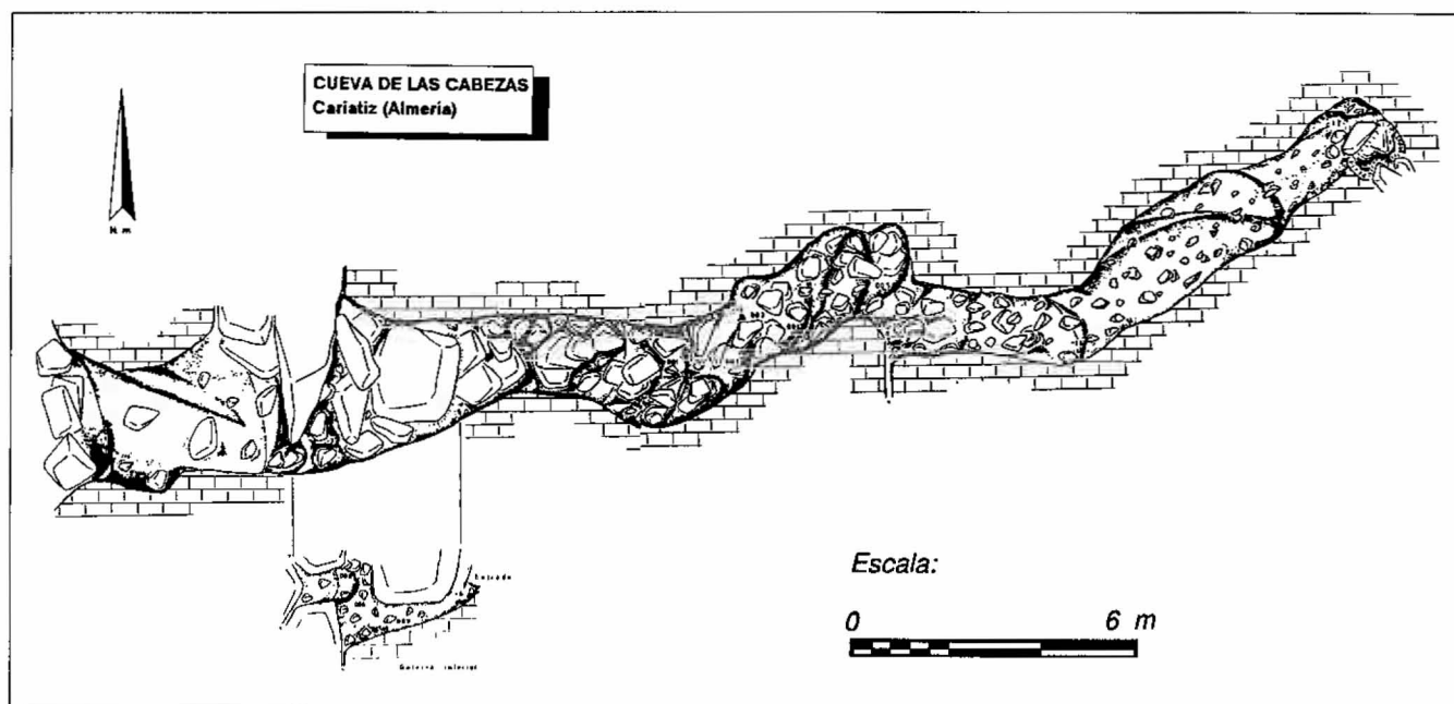
Figura 3 Cueva de las Cabezas (Cariatiz, Almería). Topografía: (F. Risco, SECAM)
