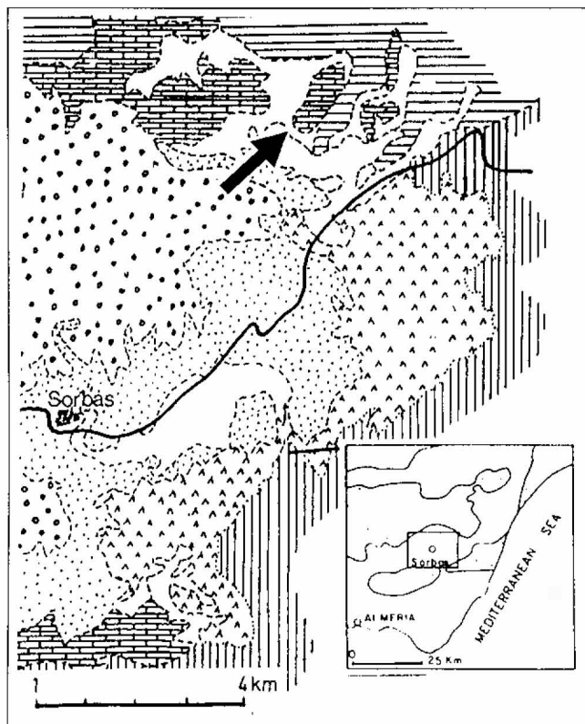
Figura 1 Situación del afloramiento arrecifal de Cariatiz (Almería) (modificado de PULIDO BOSCH y CALAFORRA, 1993)
